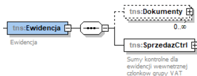
Diagram 5. The structure of the element Ewidencja of JPK_GV
