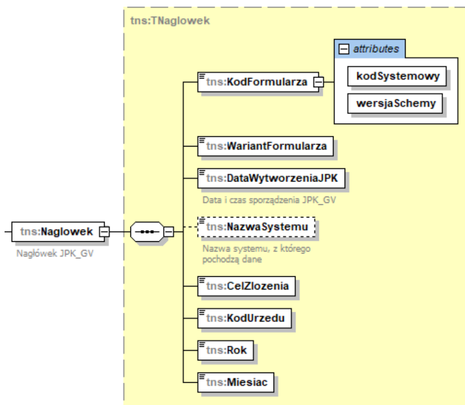
Schemat 2. Struktura elementu Naglowek dla JPK_GV
