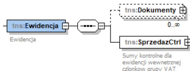
Schemat 5. Struktura elementu Ewidencja dla JPK_GV
