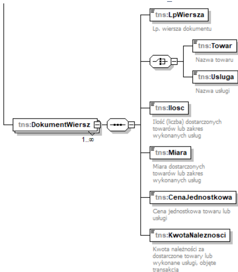
Schemat 7. Struktura elementu DokumentWiersz dla JPK_GV
