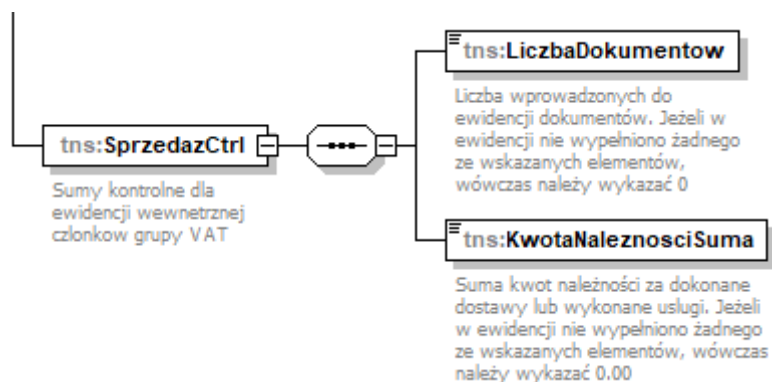
Schemat 8. Struktura elementu SprzedazCtrl dla JPK_GV
