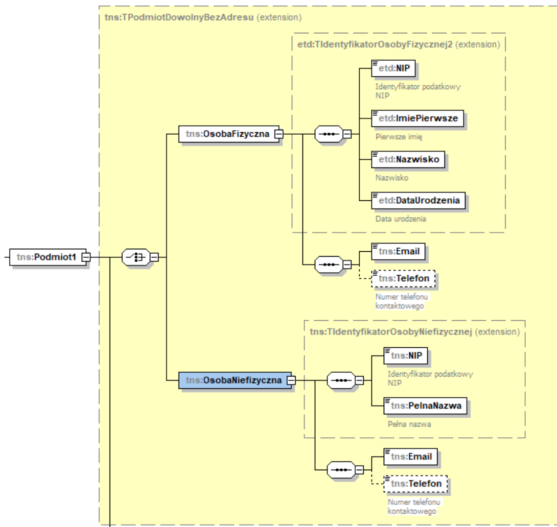
Schemat 3. Struktura elementu Podmiot1 dla JPK_GV
