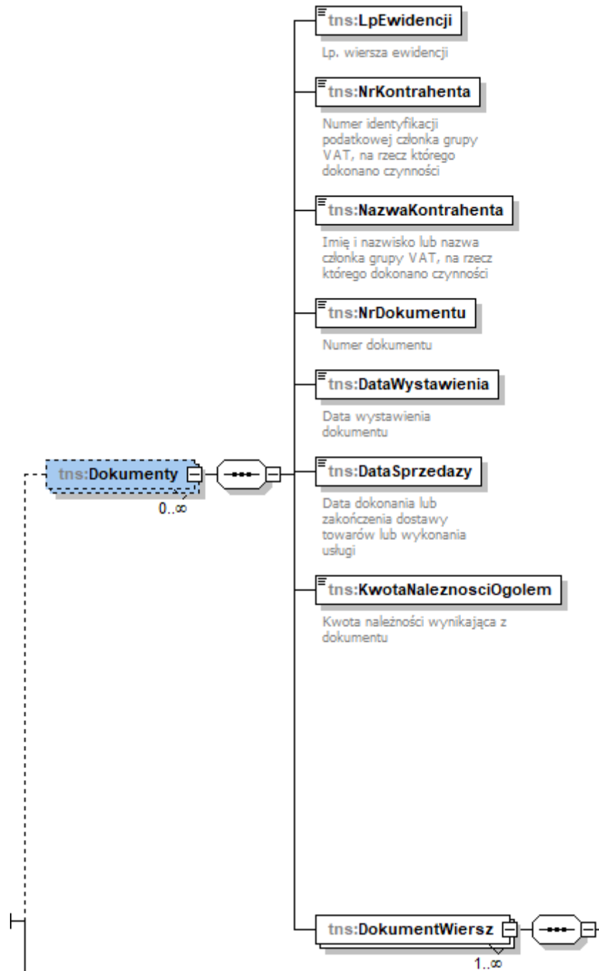
Schemat 6. Struktura elementu Dokumenty dla JPK_GV
