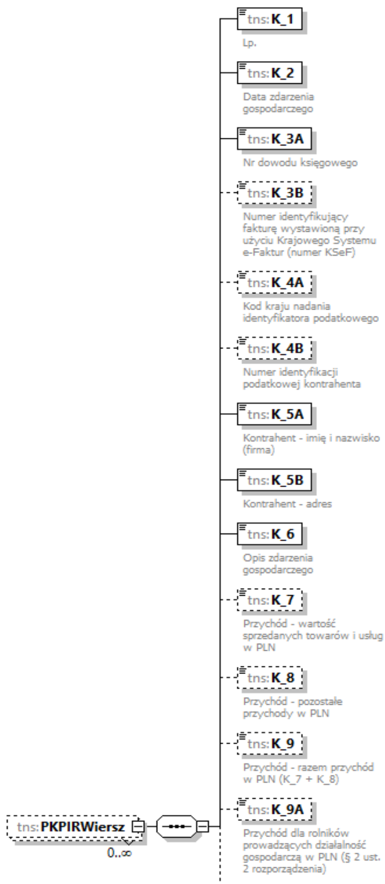
Schemat 8. Struktura węzła PKPIRWiersz.
