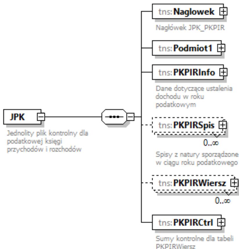
Schemat 1. Struktura JPK_PKPIR.
