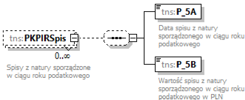
Schemat 7. Struktura węzła PKPIRSpis.
